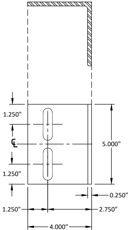
81 JAMB/HORIZONTAL 6063-T5
