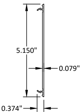
FLUSH FILLER 6063-T5
